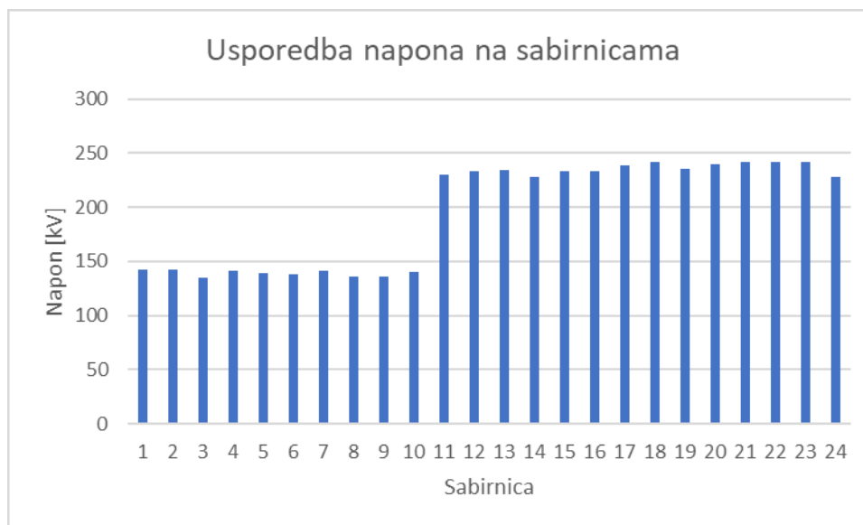
Slika 6.5. Usporedba napona na sabirnicama -scenarij 3
