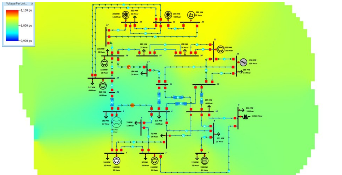
Slika 6.4. Simulirani napon u sustavu obojan pomoću funkcije contouring za scenarij 2
