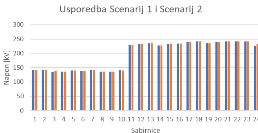
Slika 6.17. Usporedba napona scenarija 1 i scenarija 2
