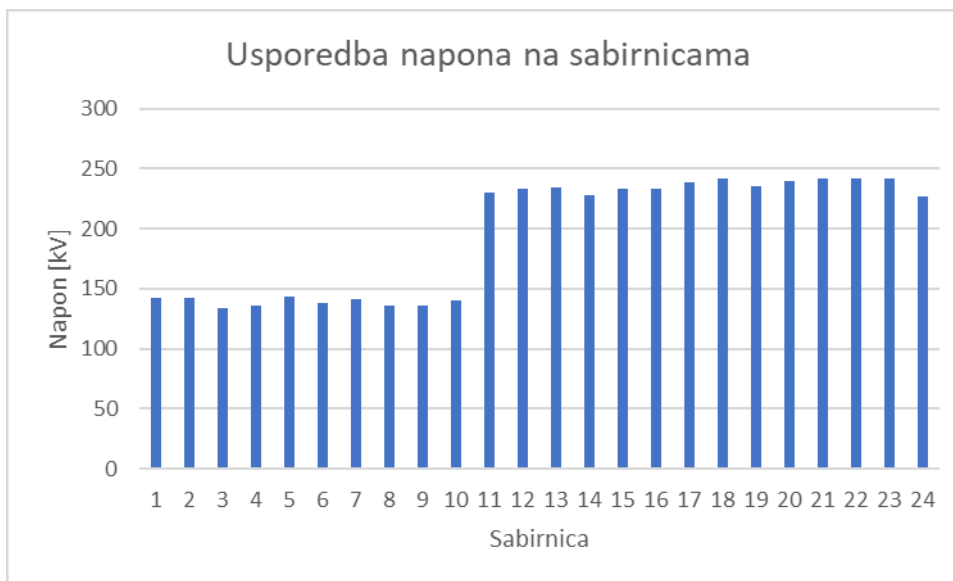
Slika 6.7. Usporedba napona na sabirnicama - scenarij 4
