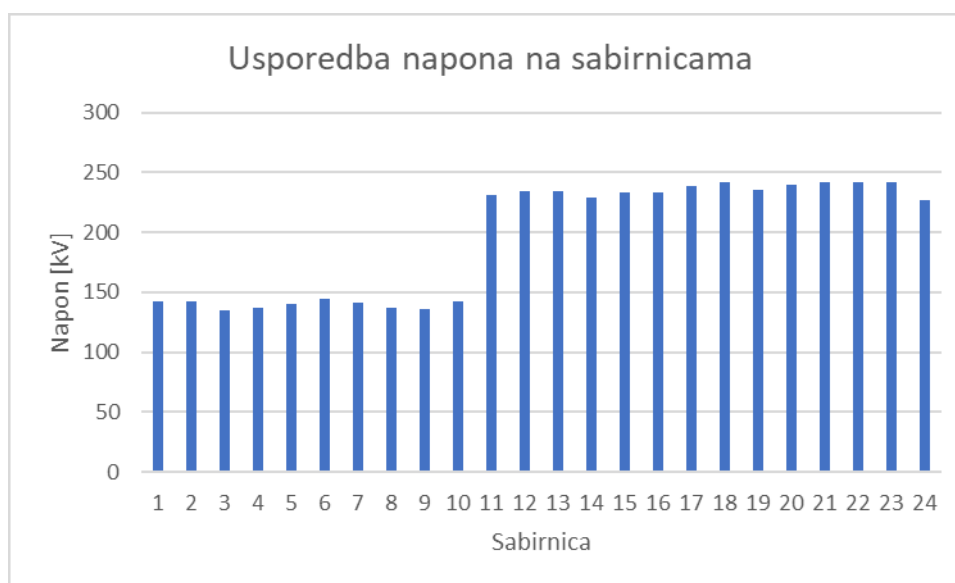
Slika 6.9. Usporedba napona na sabirnicama - scenarij 5
