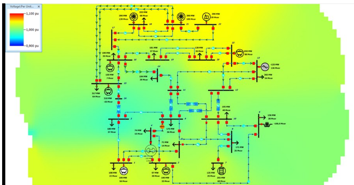
Slika 6.6. Simulirani napon u sustavu obojan pomoću funkcije contouring za scenarij 3
