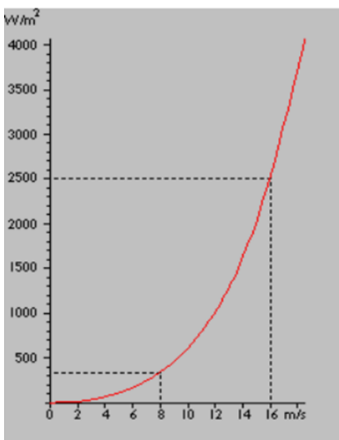
Slika 3.4. Porast snage vjetra sa brzinom [14]
