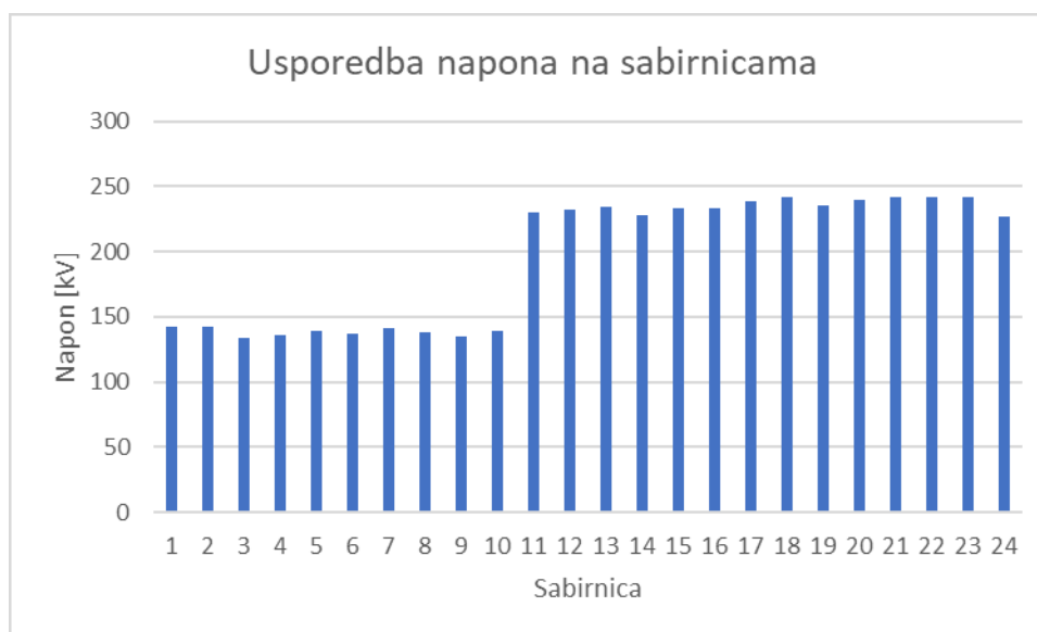
Slika 6.11. Usporedba napona na sabirnicama - scenarij 6
