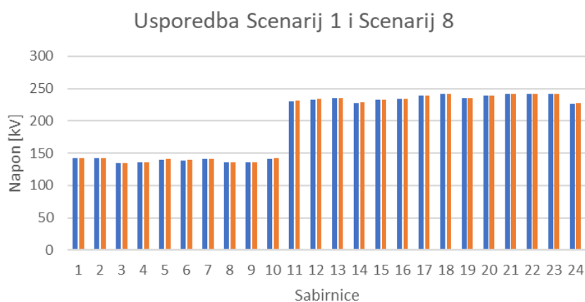
Slika 6.23. Usporedba napona scenarija 1 i scenarija 8
