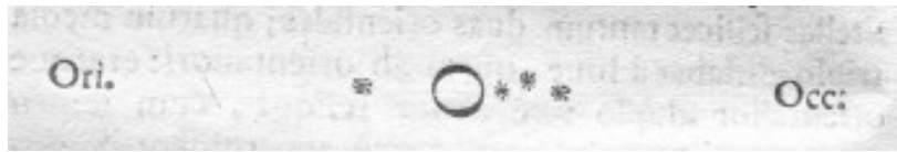
Sl. 5.12. Pozicija zvijezda u odnosu na Jupiter 13. siječnja 1610. [13].
