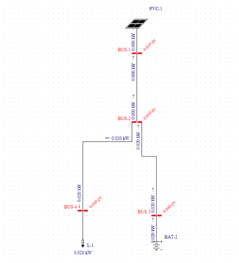
Slika 4.5 Prikaz tokova snaga
