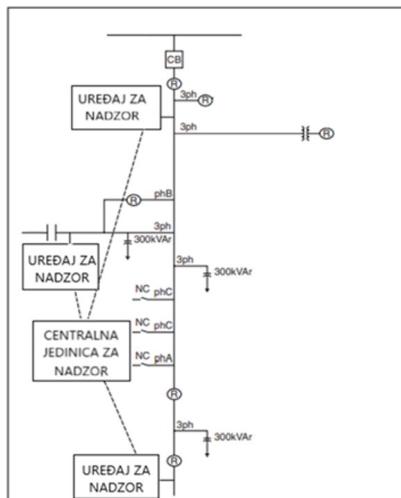
Slika 3.1 Prikaz nadzora kvalitete električne energije napojne mreže [1]
