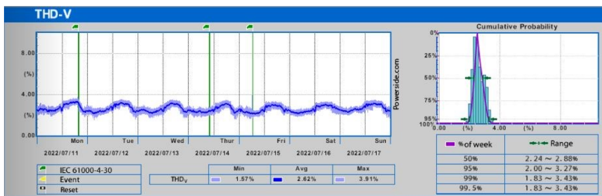
Slika 5.3 Dijagram THD-V
