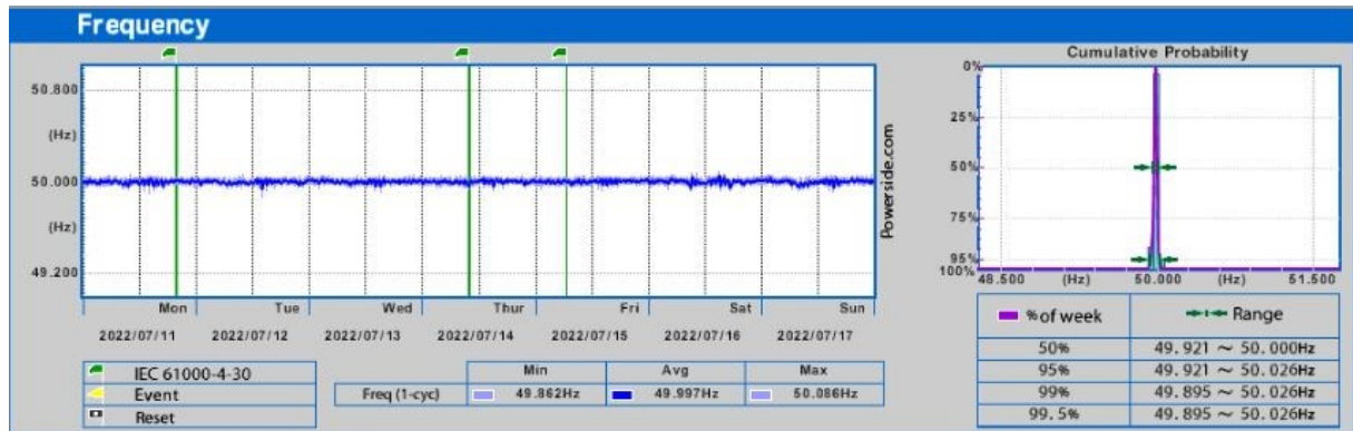
Slika 6.4 Dijagram frekvencije
