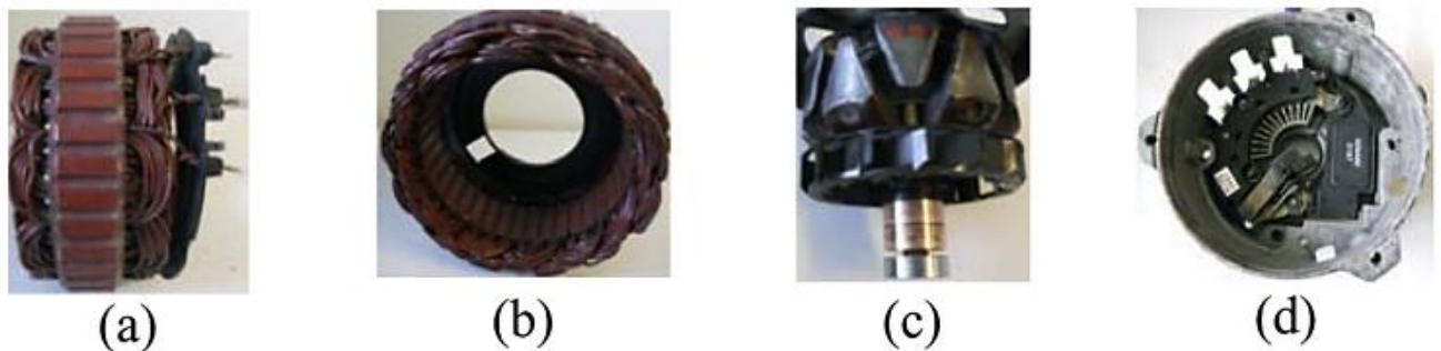
Slika 6.6 Standardni dijelovi automobilskeg alternatora sa kandža kavezom na rotoru; (a) i (b) stator sa zubcima i utorima, (c) rotor, (d) energetskeg elektronika [21]
