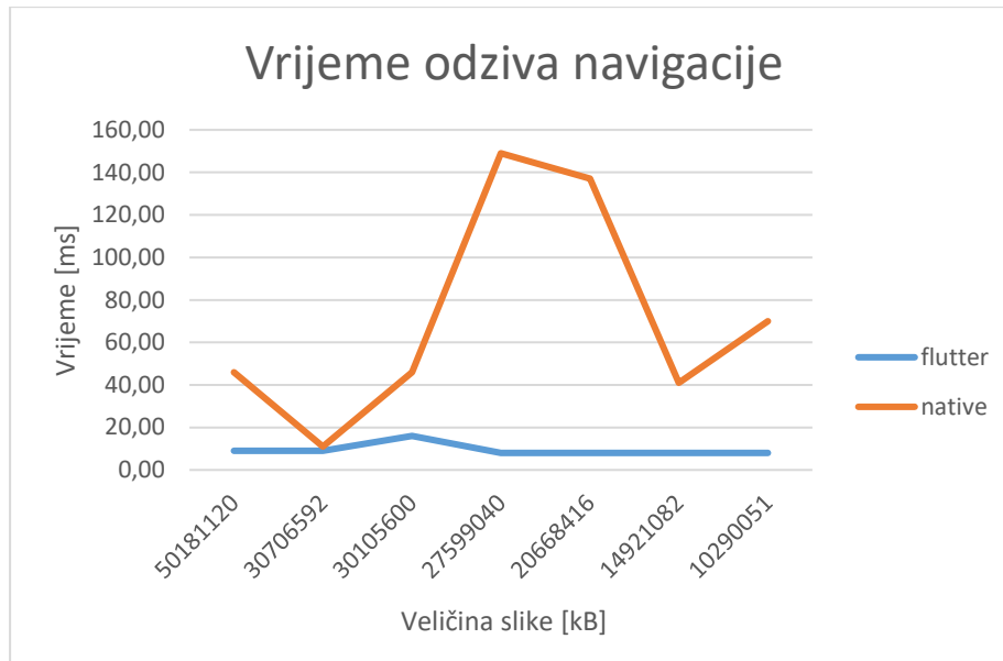
Slika 5.2. Vrijeme odziva navigacije iPhone 13 Pro Max
