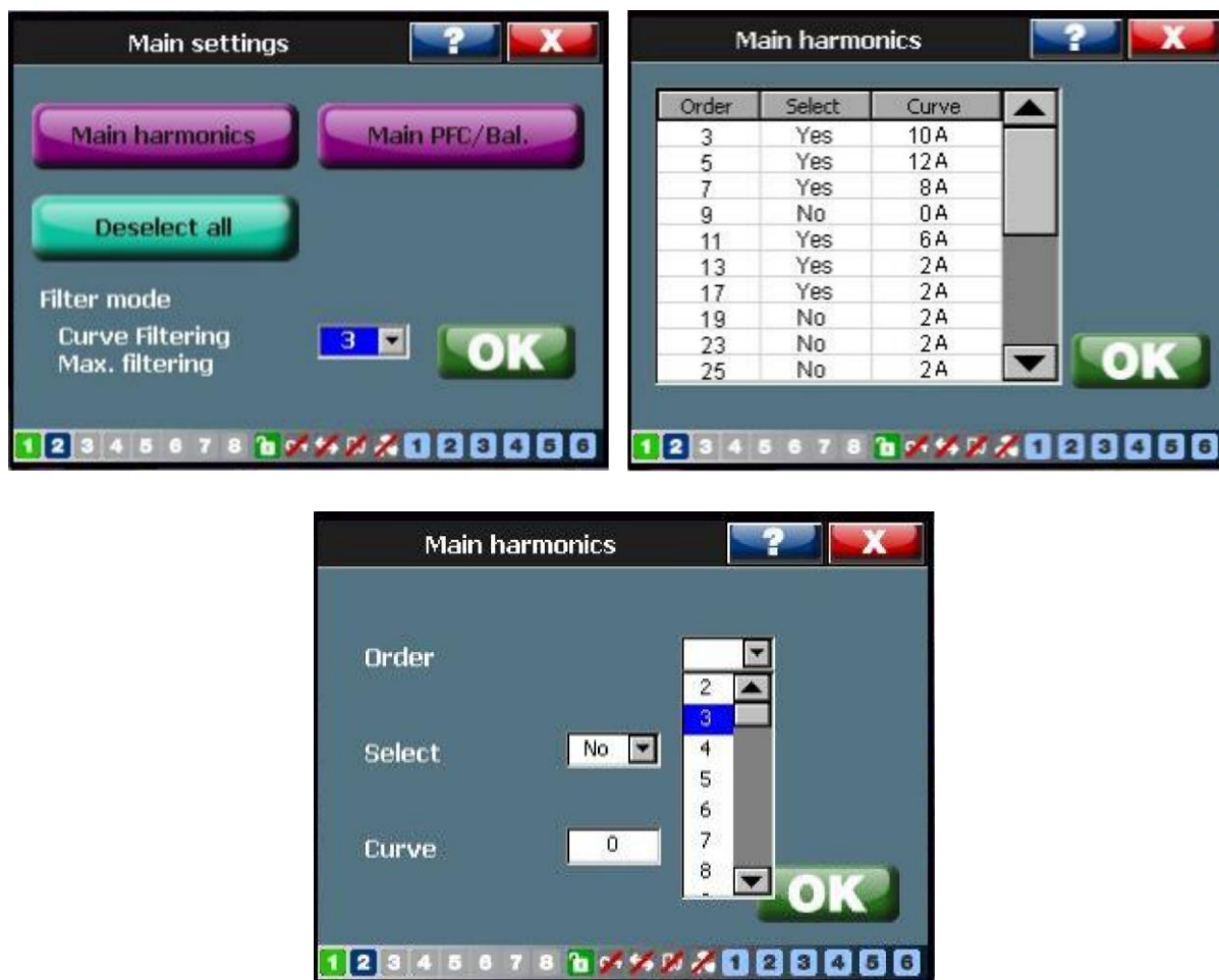
Slika 4.8. Podešavanje harmonika [29]
