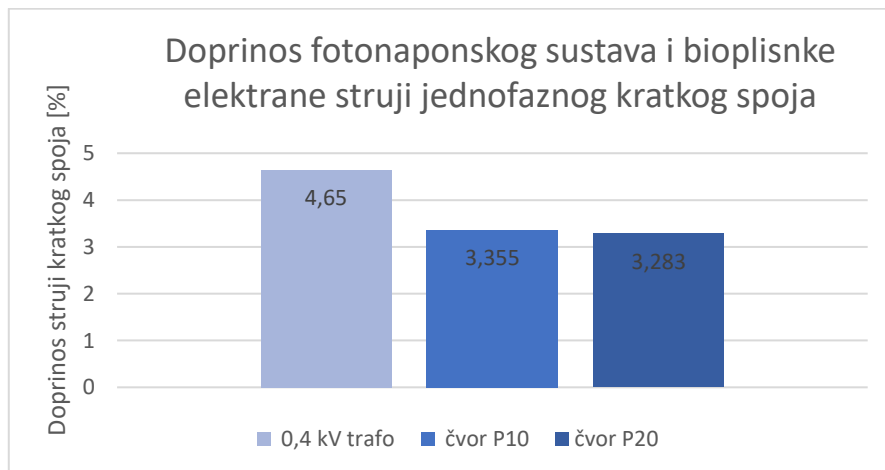
Grafikon 6.10. Doprinos fotonaponskog sustava i bioplinske elektrane struji jednofaznog kratkog spoja
