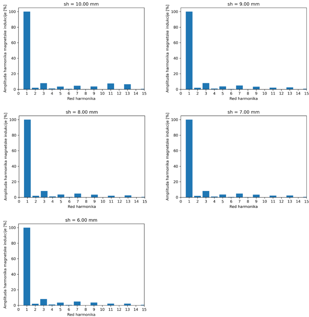
Slika 5.20. Spektralni sastav signala magnetske indukcije pri promjeni visine udara statora
