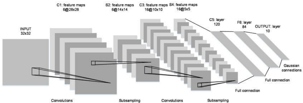
Slika 2.6. LeNet-5 arhitektura 6
