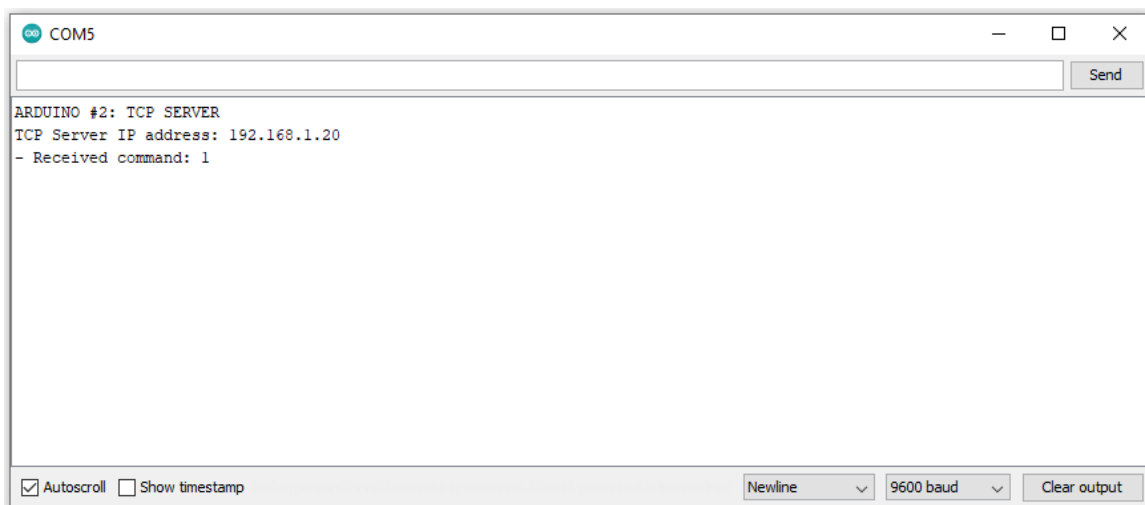
Slika 3.7. Arduino server Serial Monitor
