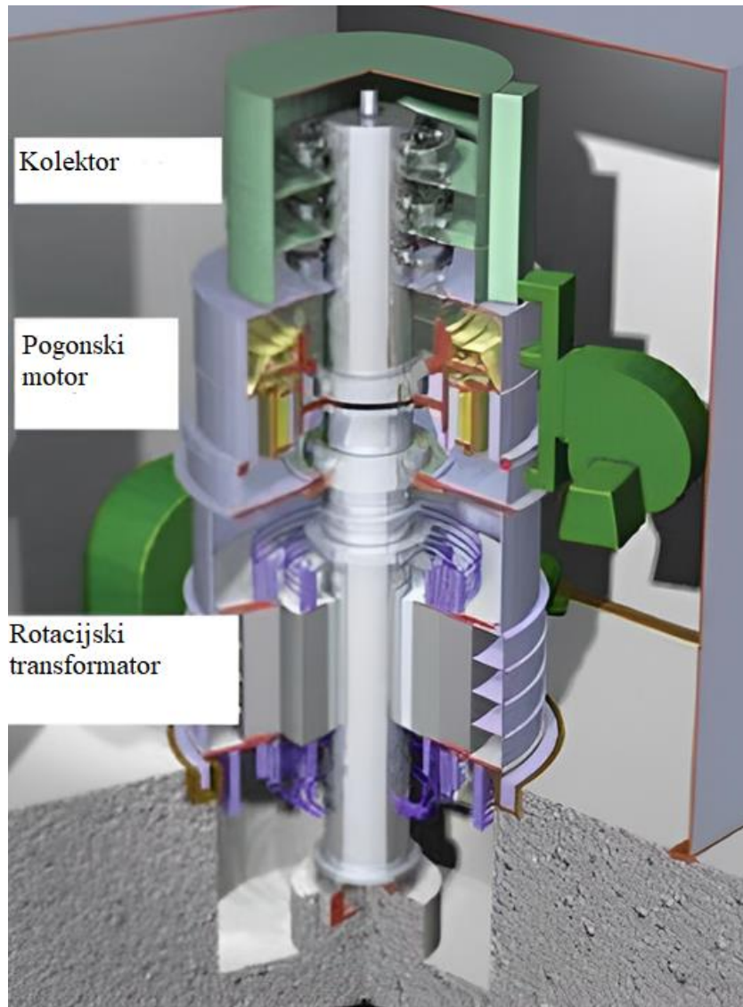
Slika 3.1. Dijelovi VFT-a [6]
