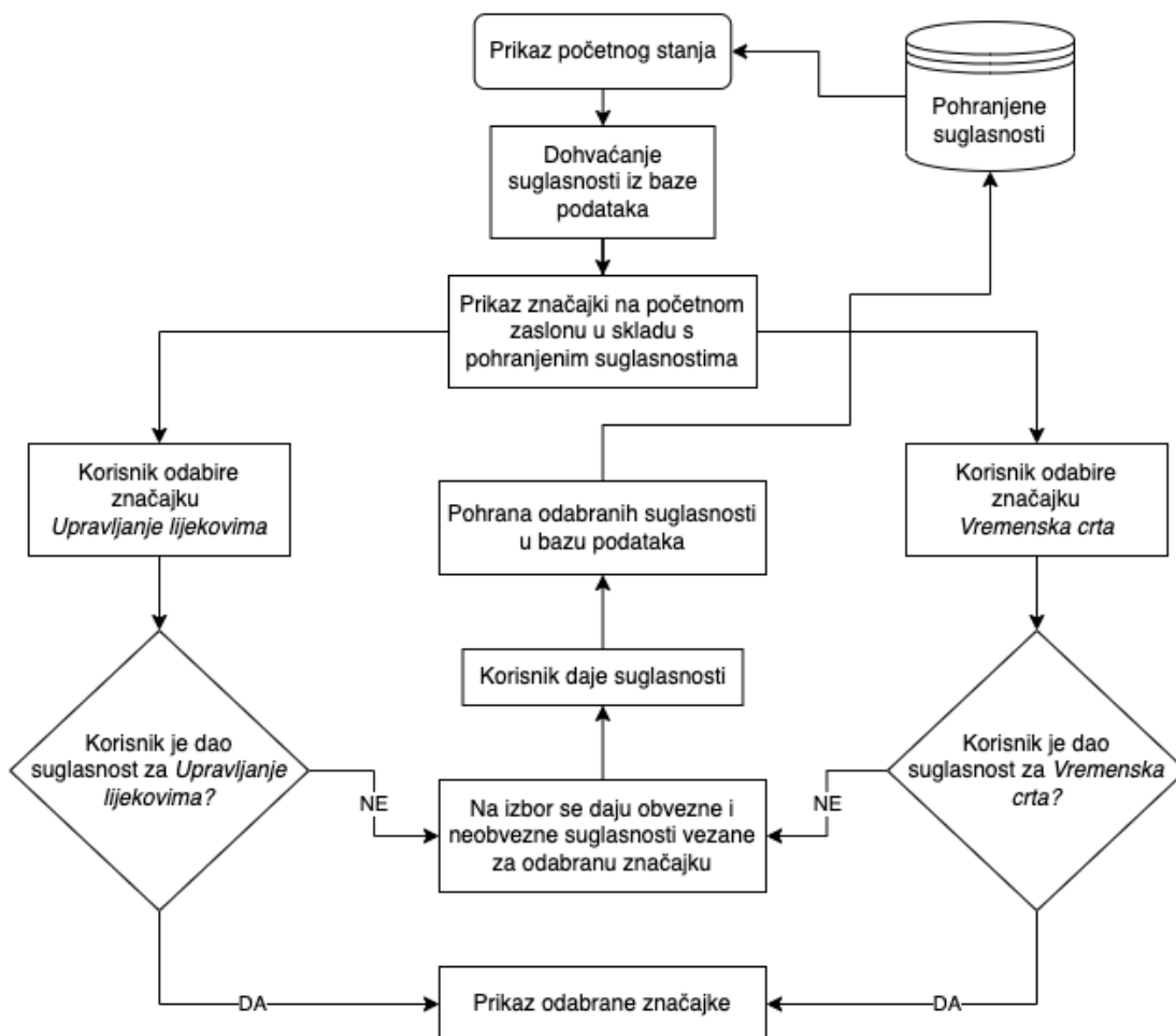
Sl. 4.1. Dijagram tjeka značajke za upravljanje suglasnostima
