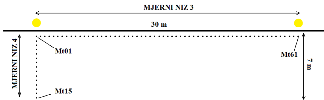
Sl. 4.11. Skica mjerenja na šetnici
