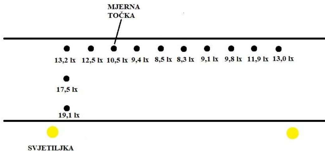
Sl. 4.7. Rezultati mjerenja rasvijetljenosti na prometnici prema normi HRN EN 13201-3:2016
