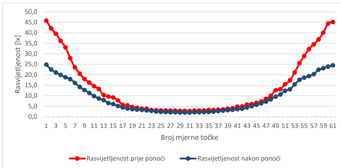
Sl. 4.13. Rasvjetljenost uzduž šetnice (mjerni niz 1), prije i nakon ponoći
