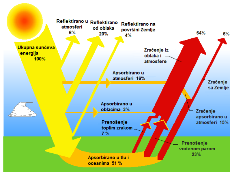
Sl.2.1. Zemljina energetska bilanca [2]
