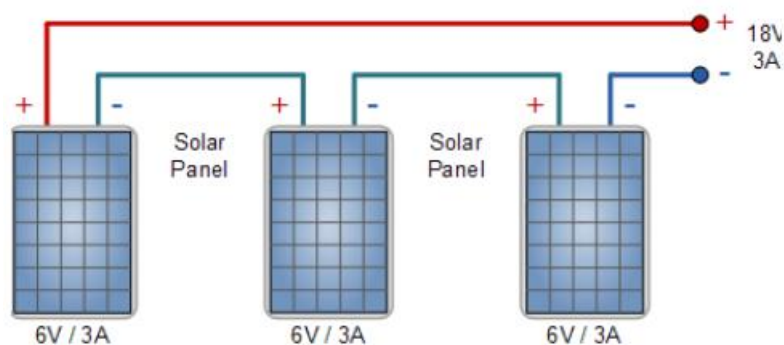
Sl. 2.6. Serijski spoj fotonaponskih modula, izvor kao [1]
