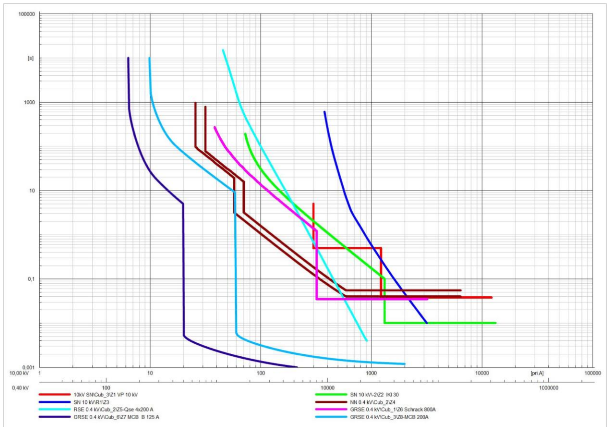
Slika 4.11. Isklopne karakteristike
