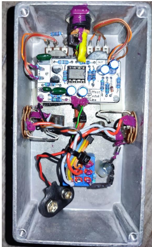
Slika 5.3: Unutrašnjost fizičkog modela pedale
