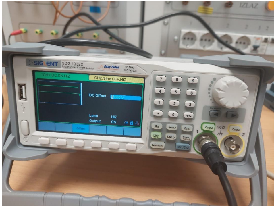
Slika 4.17 Funkcijski generator
