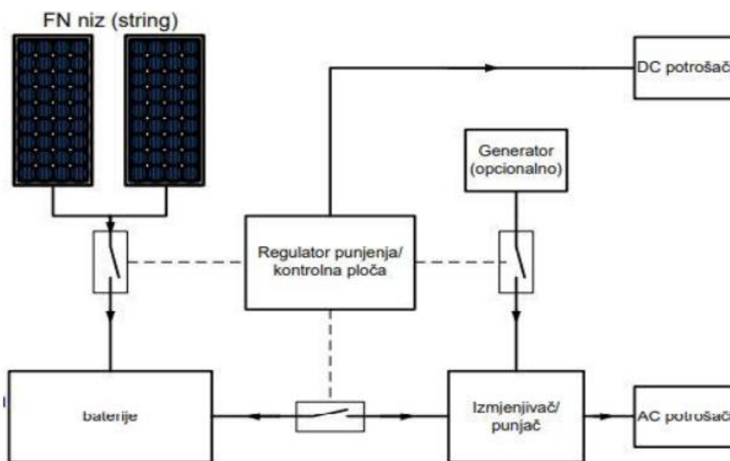
Slika 3.14. Prikaz autonomnog (off-grid) fotonaponskog sustava [3]
