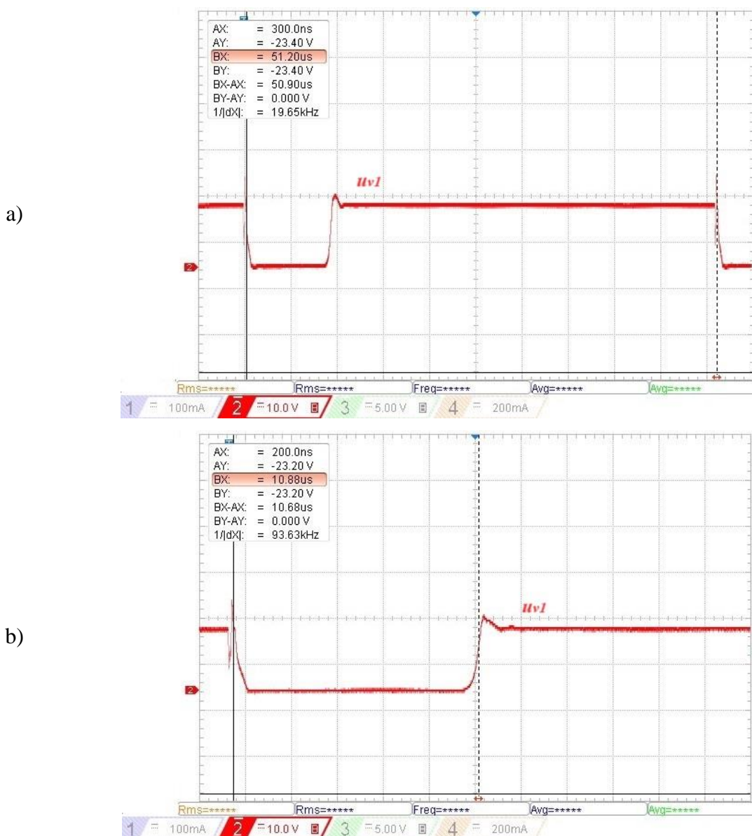
Slika 5.3. Mjerenje: a) sklopne periode, b) vremena vođenja MOSFET-a
