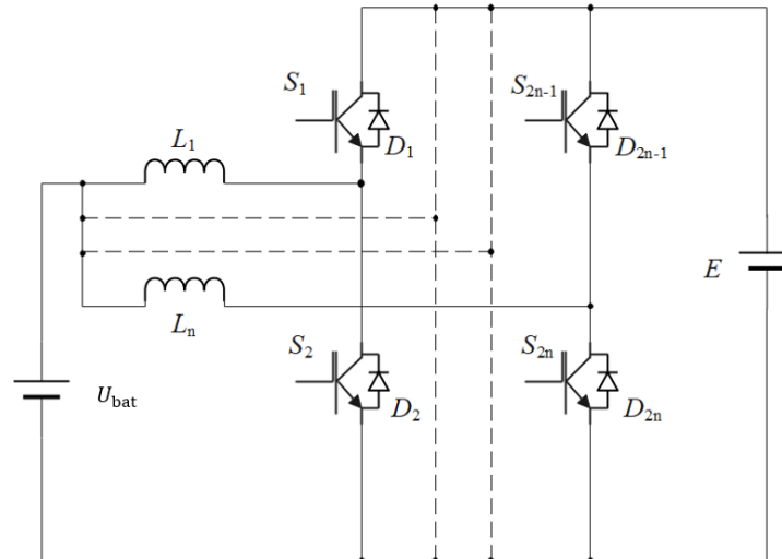
Slika 4.1. Nadomjesna shema dvosmjernog istosmjernog pretvarača s n grana
