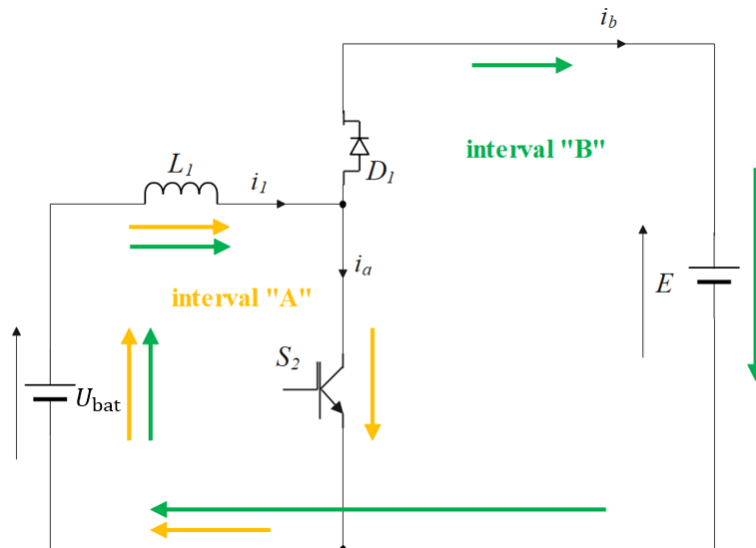
Slika 4.6. Izvedena nadomjesna shema za uzlazni režim rada jedne grane
