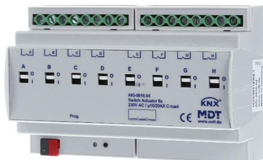
Slika 3.7. : MDT AKI-0816.04 Aktuator sklopki/prigušivač rasvjete [38]
