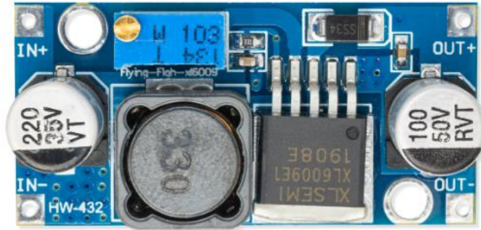
Sl. 2.5. Prikaz pretvarača napona s XL6009
