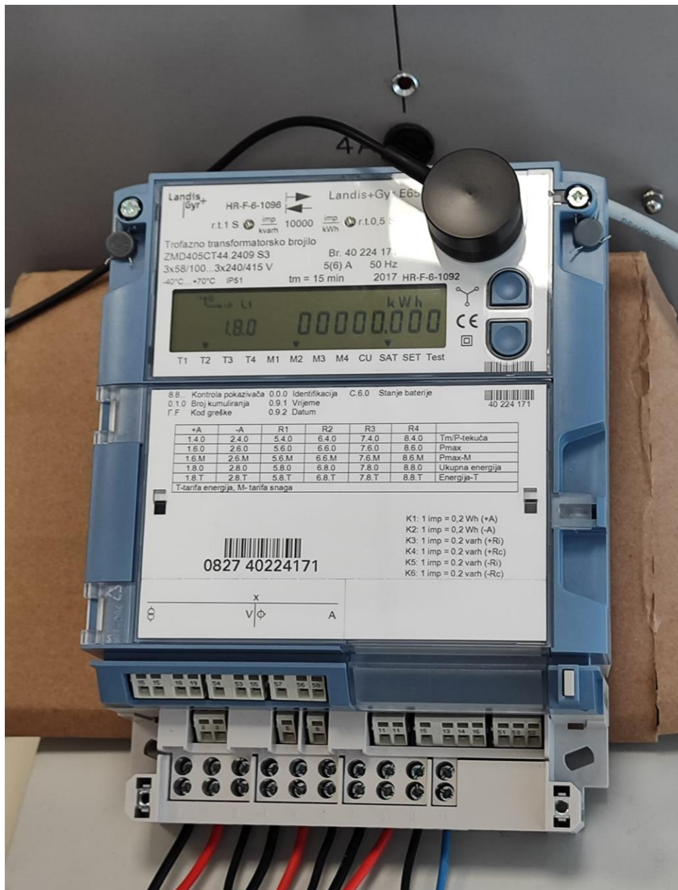
Slika 3.1. Landis+Gyr ZMD405CT44 brojilo električne energije
