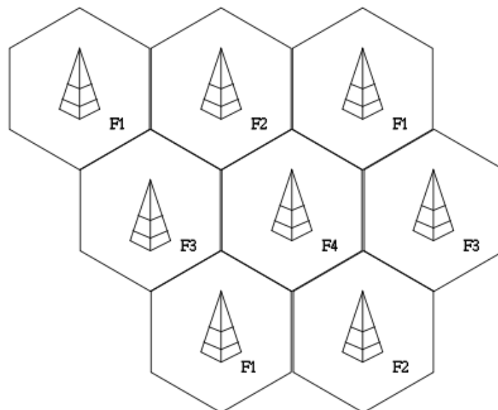
Slika 4.14. Cellular mreža
