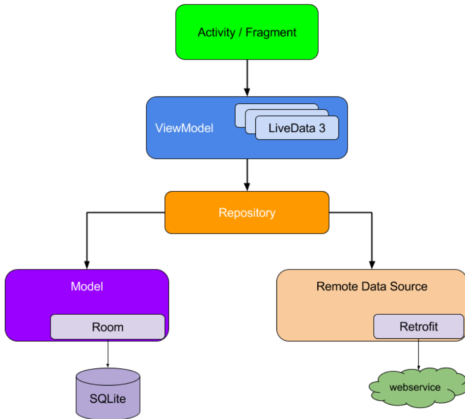
Slika 3.3. MVVM arhitektura [4]
