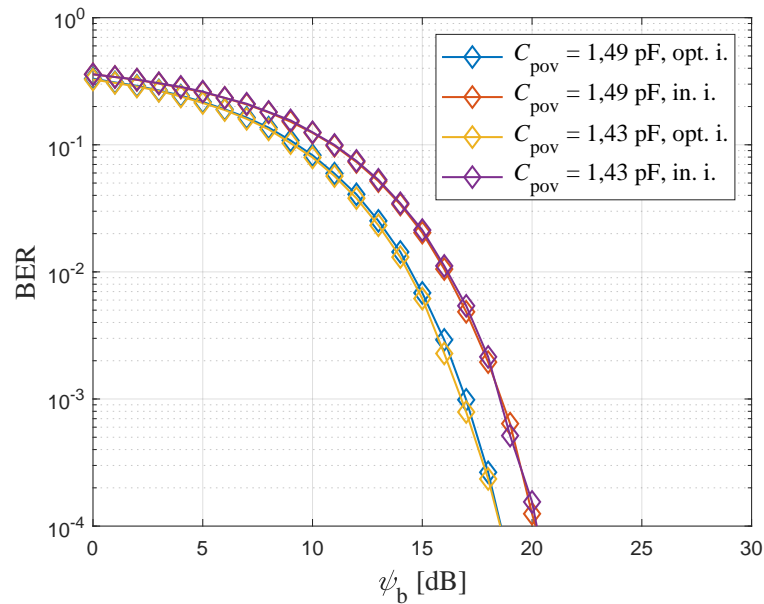
Slika 4.19: Učestalost pogreške prilikom detekcije bita (BER) kod ISK-CC-HBC uz C_{\text{pov}} = 1,49 [pF] i C_{\text{pov}} = 1,43 [pF]
