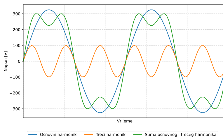
Slika 2.1. Osnovni valni oblik struje i izobličen oblik trećeg harmonika
