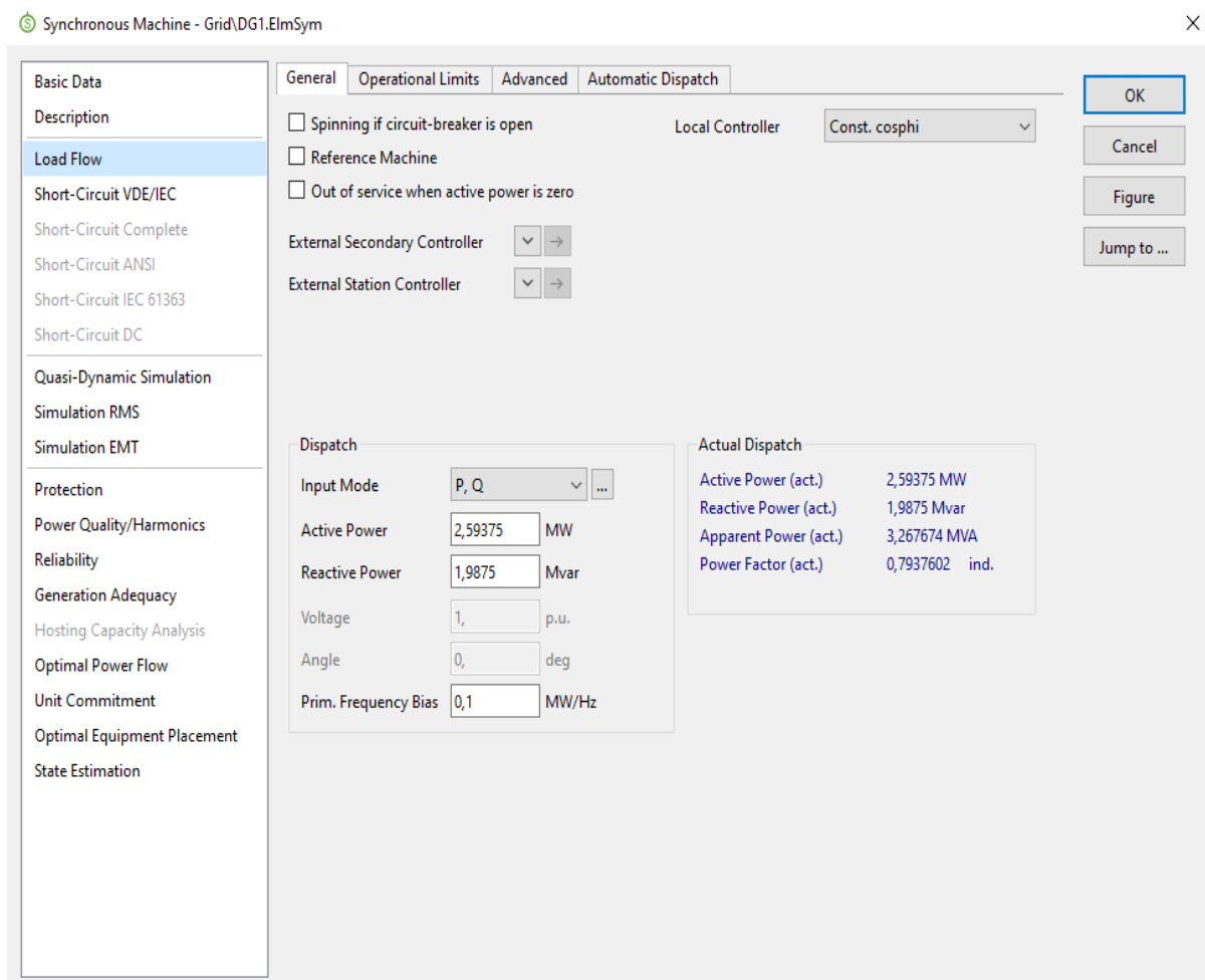
Slika 4.40. Podaci DG1 u slučaju kad je proizvodnja veća od potrošnje
