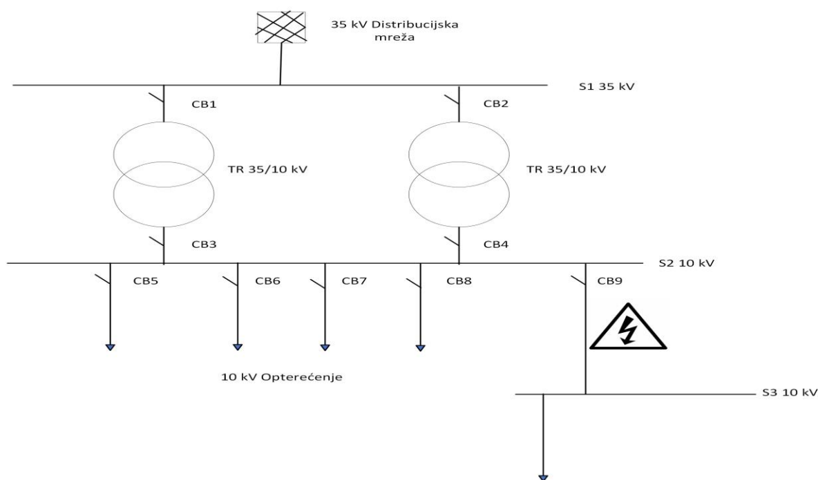
Slika 3.1. Distribucijska mreža
