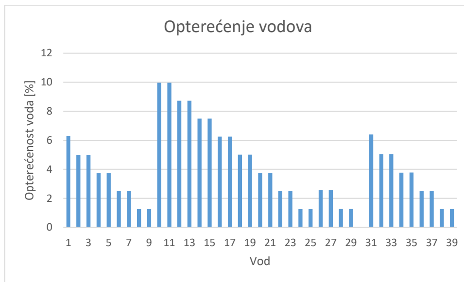
Slika 6.11. Prikaz opterećenosti pojedinog voda
