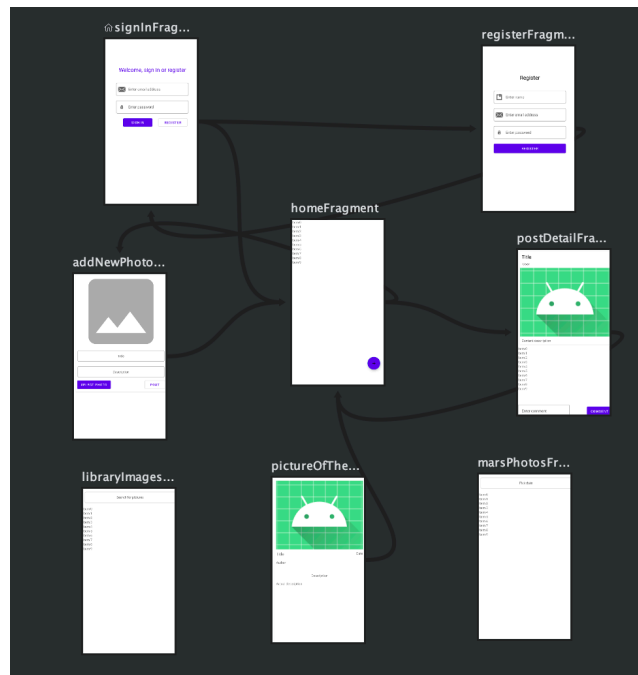
Slika 3.18. Navigacijski graf
