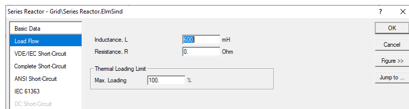
Slika 5.6: Podešenje parametara serijskih prigušnica: L = 600 mH, R = 0 \Omega
