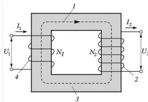
Slika 2.1. Shematski prikaz transformatora (1. magnetski tok, 2. sekundarni namot, 3. mag. tok, 4. primarni namot) [1]
