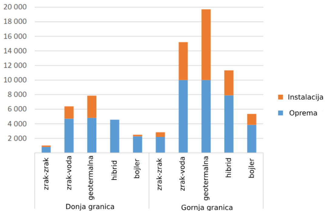
Slika 7.5. Uobičajeni početni troškovi za pojedinačne sustave grijanja u EU (u eurima) [70].
