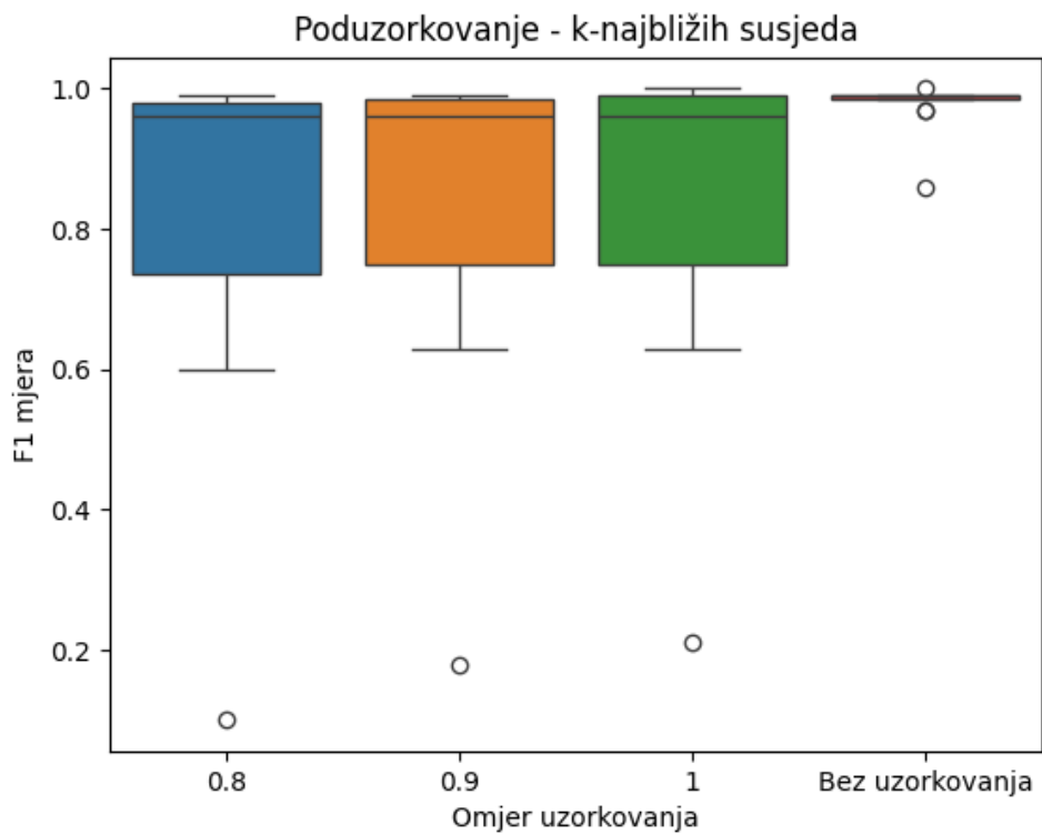
Sl. 4.12. Dijagram pravokutnika vrijednosti F1 mjere za algoritam k-najbližih susjeda pri različitom omjeru uzorkovanja
