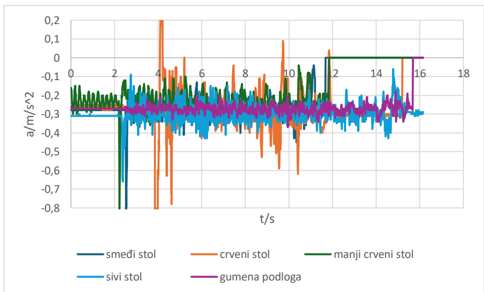
Slika 4.13. Grafički rezultati povlačenja uže strane drvene pločice
