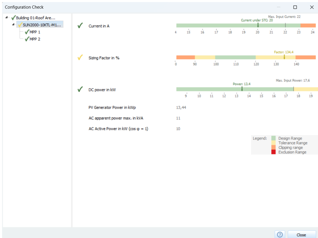
Slika 5.10. Parametri izmjenjivača
