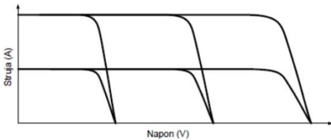
Slika 2.16. U-I karakteristika kombinirano spojenih FN modula [2]
