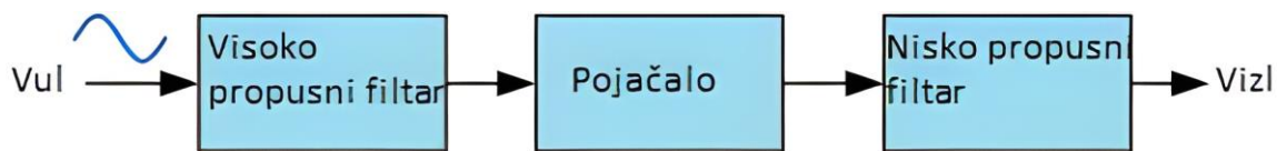
Sl. 2.3. Princip rada pojasno propusnog filtra [8]
