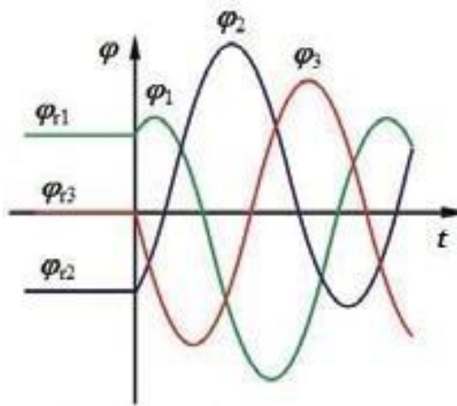
Slika 3.25. Magneticki tokovi trofaznog transformatora za povoljno odabrani trenutak uklapanja [5]
