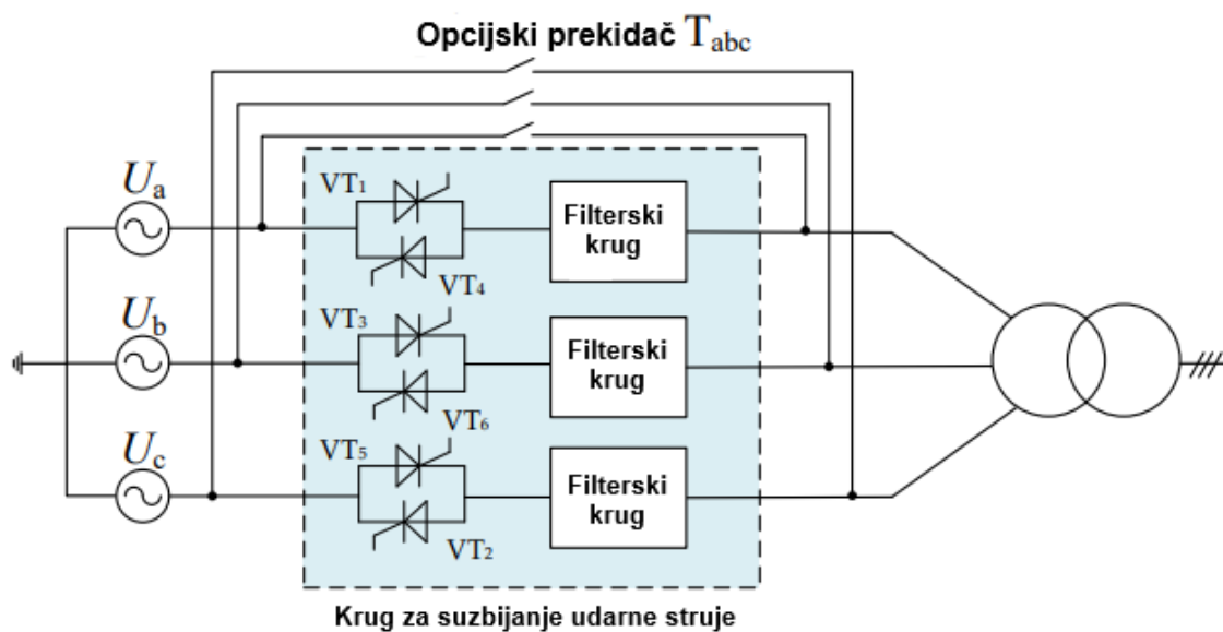
Slika 4.14. Sustav s antiparalelnim spojem tiristora s filterom [42]
