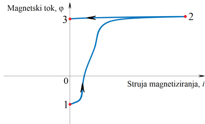
Slika 3.22. Proces predmagnetiziranja prikazan u \phi - i ravnni [19]
