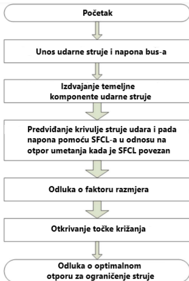
Slika 4.12. Shema za određivanje optimalne vrijednosti CLR za SFCL [39]
