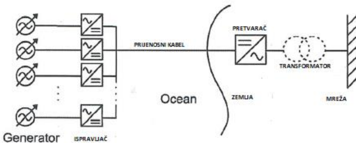
Slika 3.2. Način povezivanja više generatora na morske valove na mrežu. [25]
