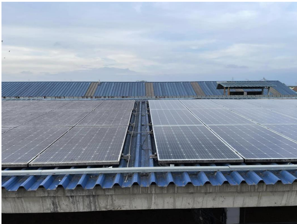
Slika 5.2 Prikaz usporedbe čistih i prljavih fotonaponskih modula
