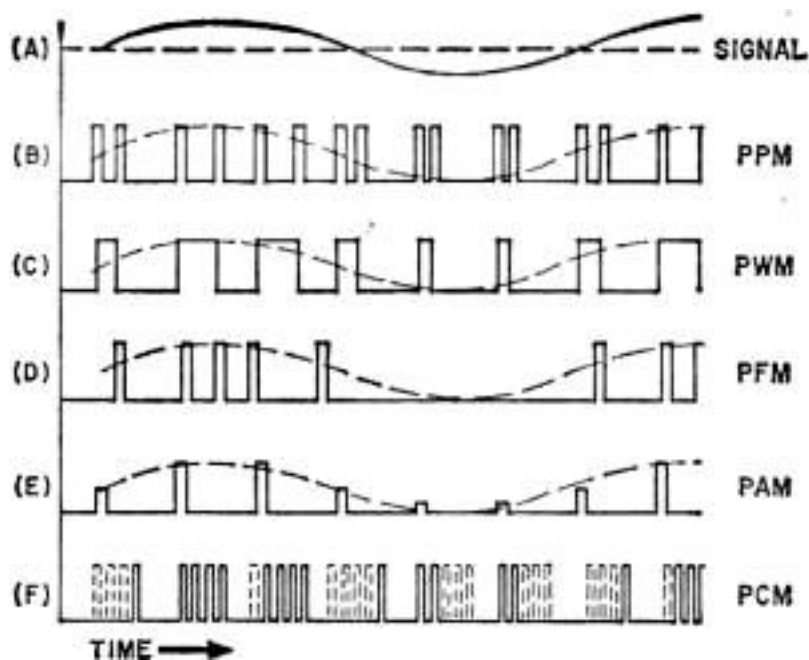
Slika 4.1 Pulsna modulacija [7]
