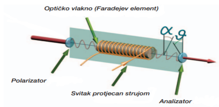
Slika 4.1.: Faradayev efekt [6]
