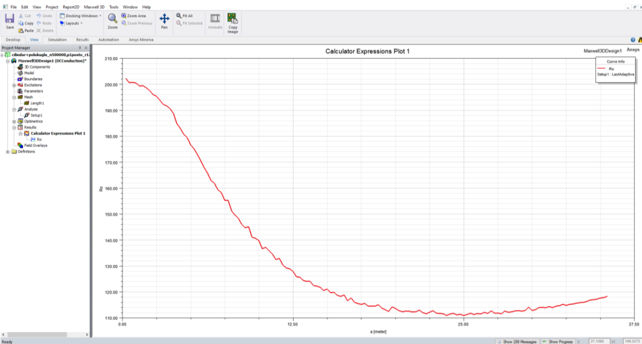
Slika 8.61. Promjena prividnog otpora tla u funkciji razmaka elektroda a , za r=120 m
