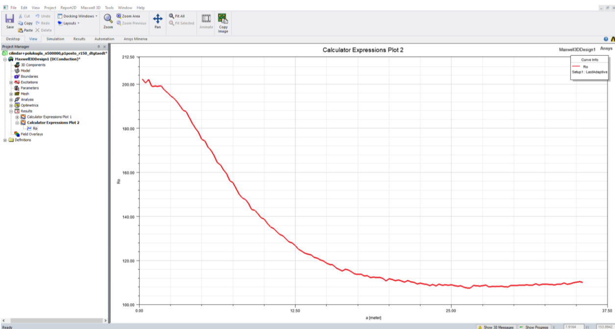
Slika 8.72. Promjena prividnog otpora tla u funkciji razmaka elektroda a , za r=150 m
