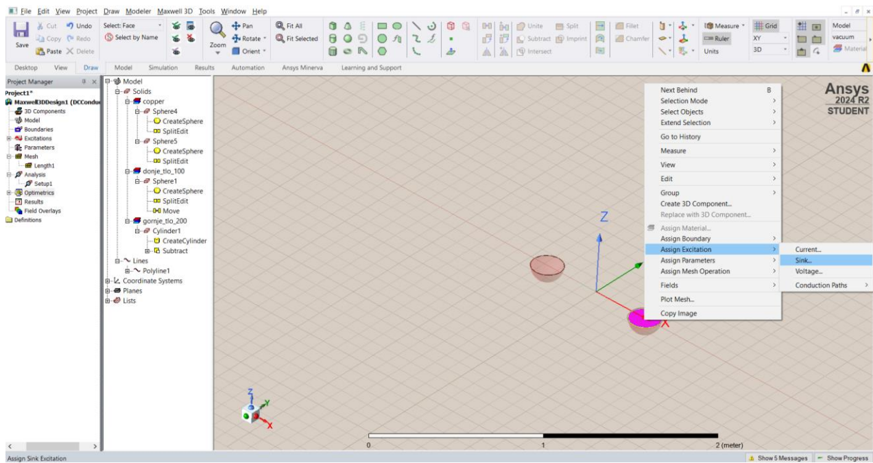
Slika 8.43. Dodavanje sink-funkcije
