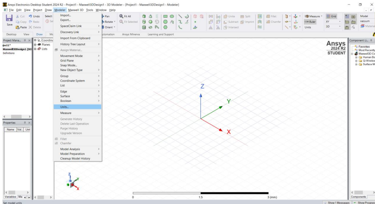
Slika 8.4. Odabir „UNITS“
