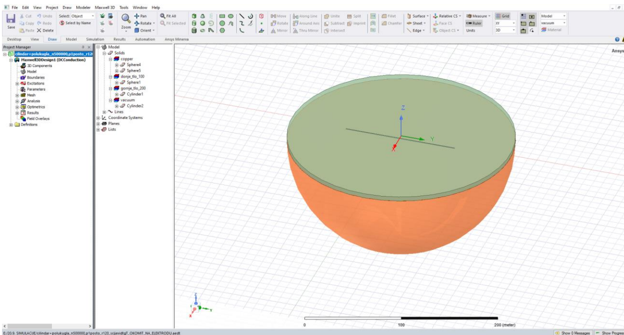
Slika 8.67. Model polukugle i cilindra za radijus 120 m, uz prisustvo okomitog cilindra u gornjem sloju tla
