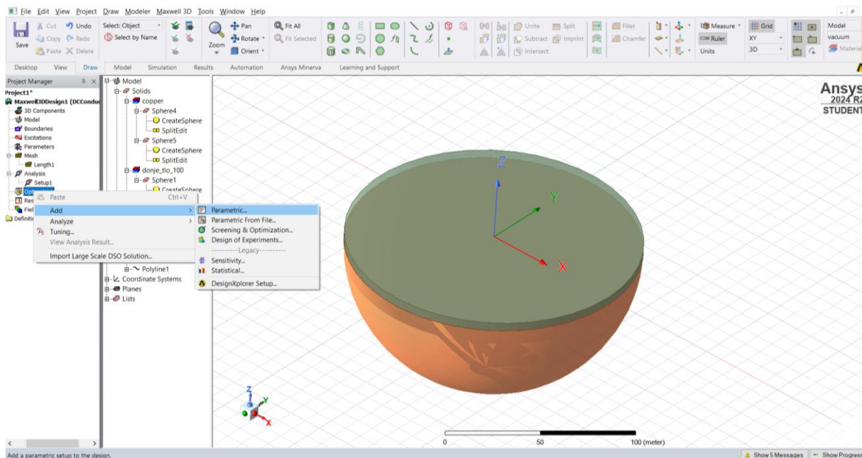
Slika 8.38. „PARAMETRIC“ funkcija
