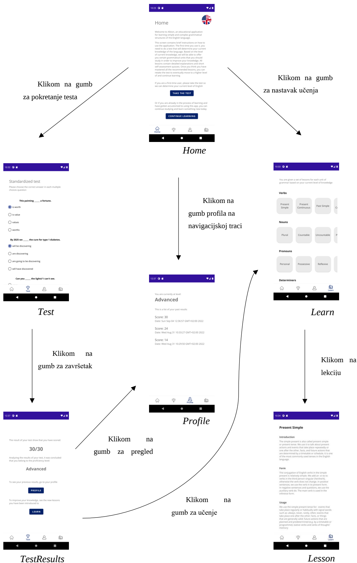
Slika 4.2 Dijagram toka aplikacije
