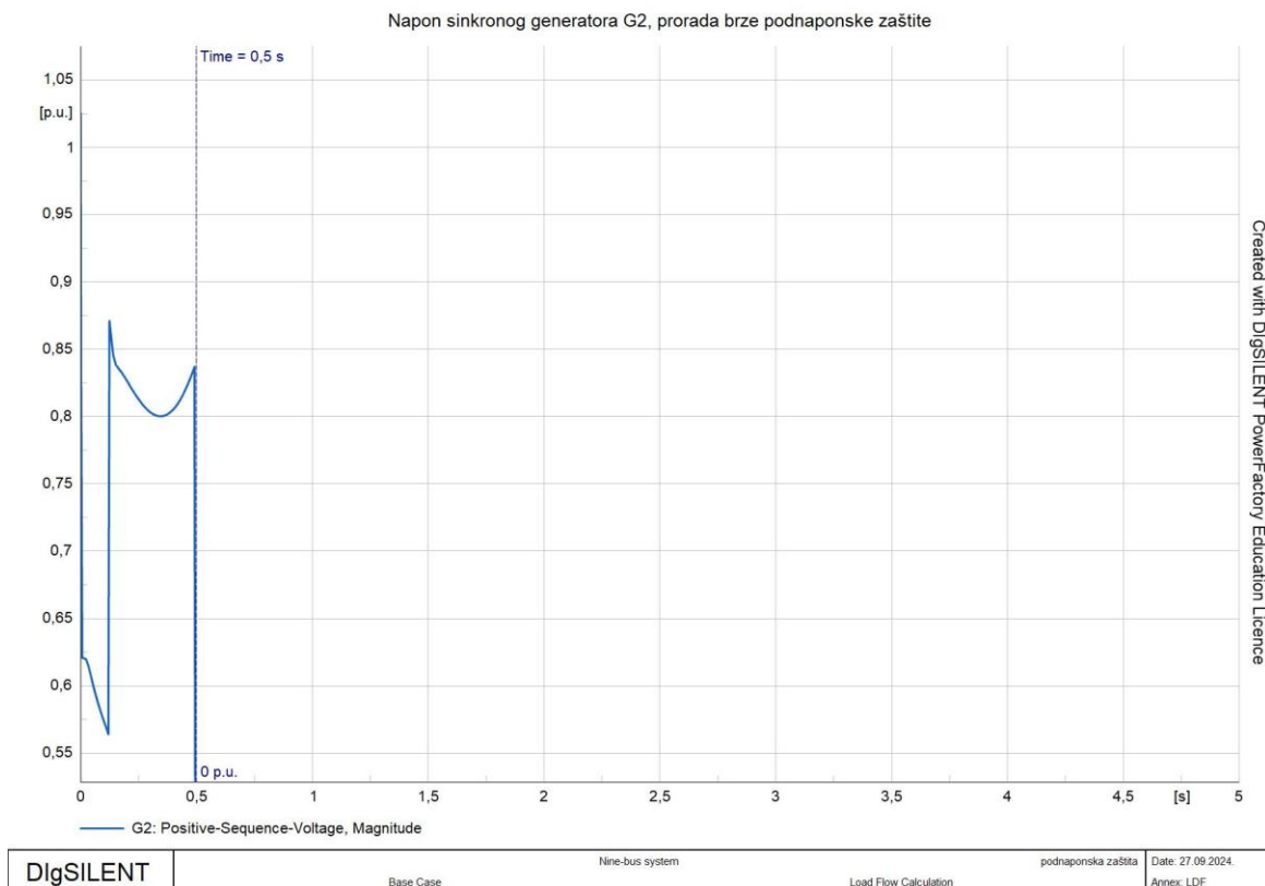
Sl. 4.6. Isključenje sinkronog generatora G2 iz mreže korištenjem brze podnaponske zaštite U_{<<}
