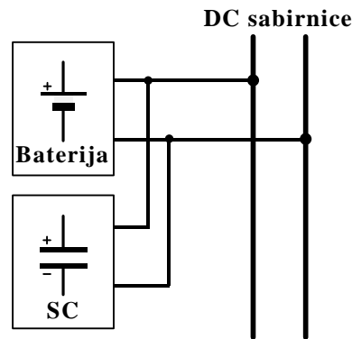
Slika 2.5. Pasivni hibridni sustav baterije i superkondenzatora (engl. passive HESS )
