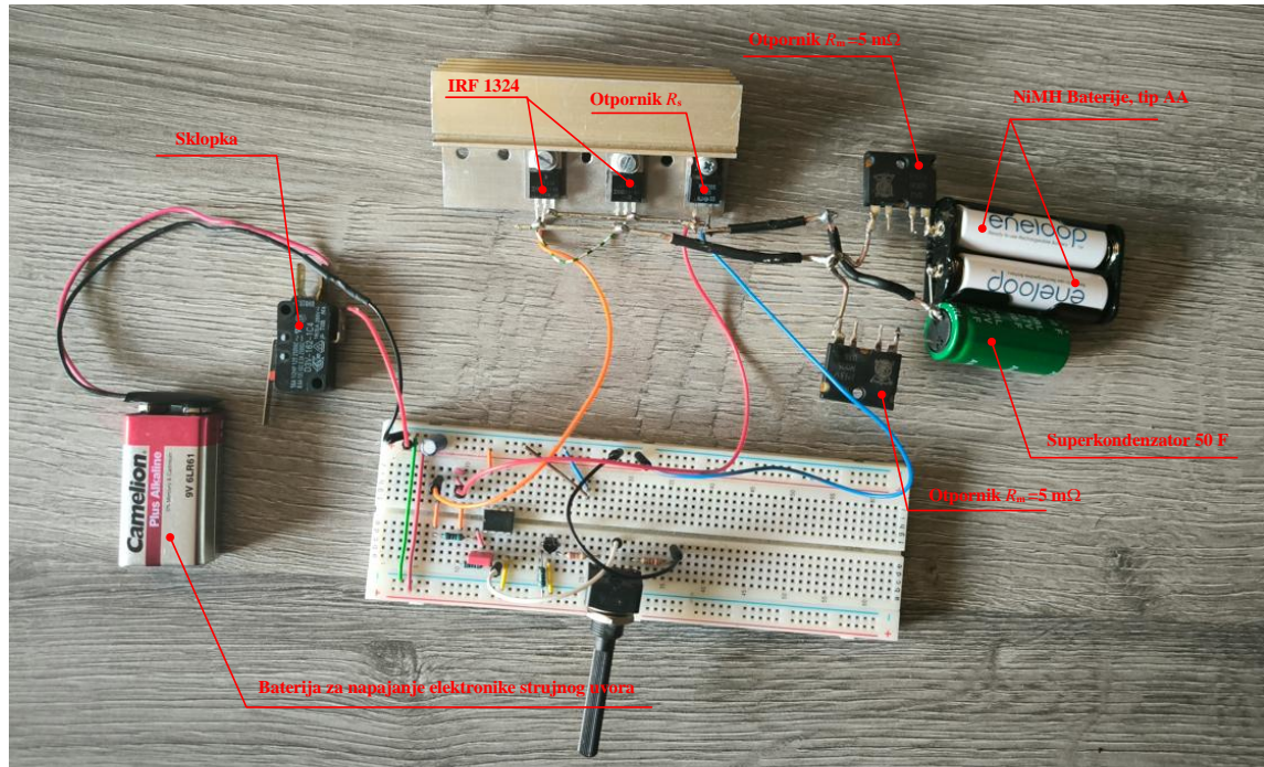
Slika 7.5. Strujni uvor, pasivni hibridni sustav baterije i superkondenzatora i mjerni otpornici
