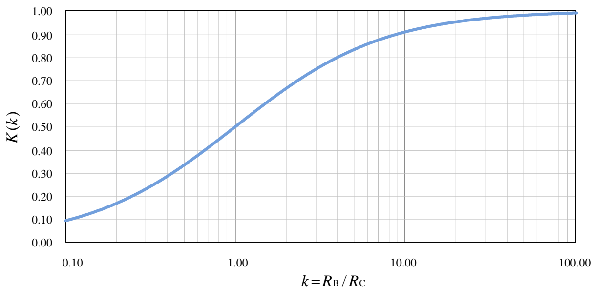
Slika 3.4. Ovisnost koeficijenta K o omjeru k = R_B / R_C
