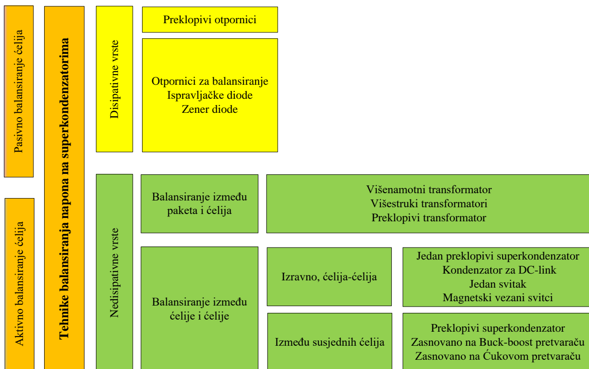
Slika 5.3. Tehnike ujednačivanja napona (balansiranja napona) na superkondenzatorima
