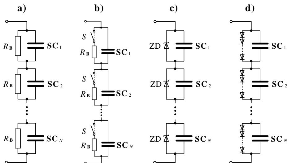
Slika 5.4. Disipativne tehnike izjednačivanja napona na superkondenzatorima, a) otpornicima, b) preklopivim otpornicima, c) zener diodama, d) ispravljačkim diodama
