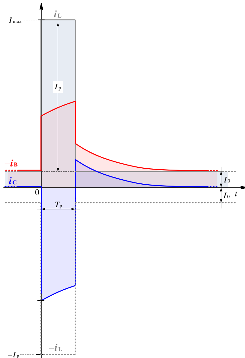
Slika 2.3. Valni oblici struje tereta, baterije i superkondenzatora
