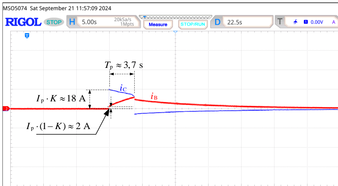
Slika 7.10. Valni oblici struja baterije i superkondenzatora izmjerenih na mjernim otpornicima ( R_m = 5 \text{ m}\Omega ) postavljenima u seriju s parom baterija i u seriju sa superkondenzatorom.
