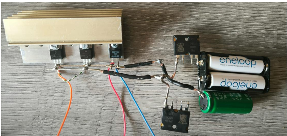
Slika 7.6. Detaljniji prikaz na HBSS i mjerne otpornike
