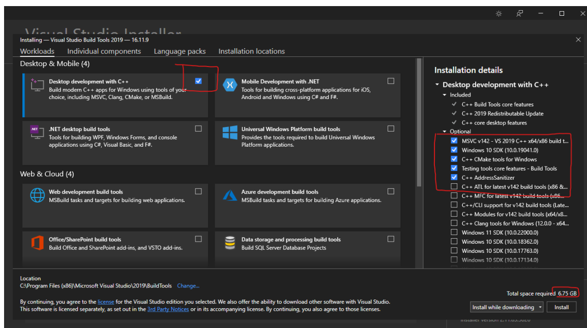
Slika 3.18: Instalacija potrebnih C++ build tools paketa
