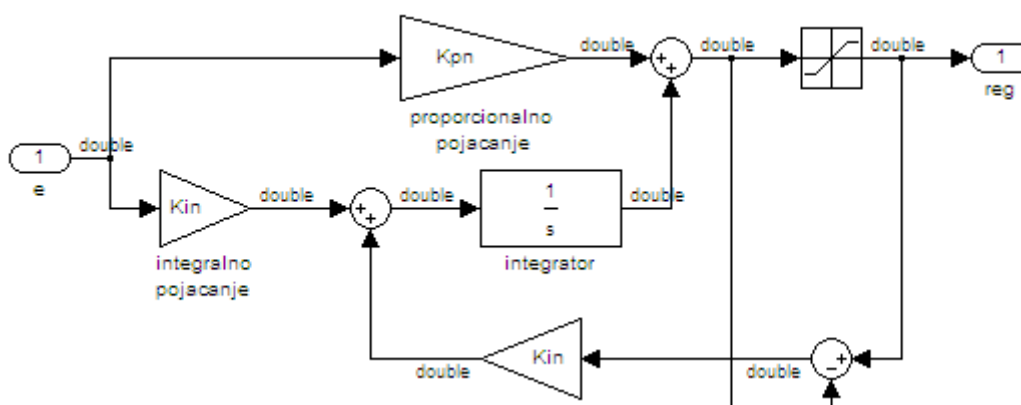
Slika 6.23. PI regulator napona sa zaštitom od zasićenja integralnog člana
