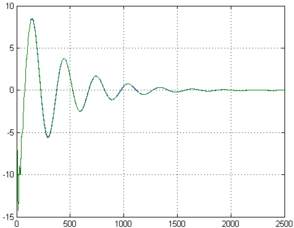
Slika 6.38. Pronyeva aproksimacija funkcije brzine vrtnje
